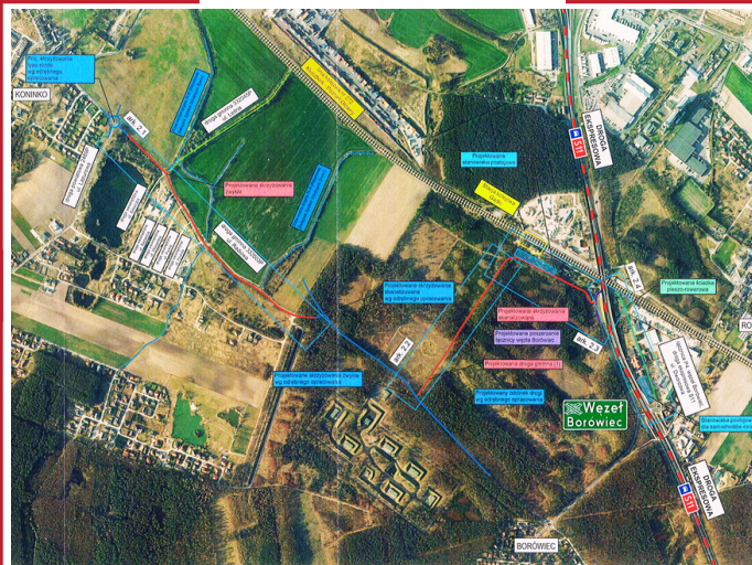
Plan budowy Węzła Przesiadkowego w Gądkach
