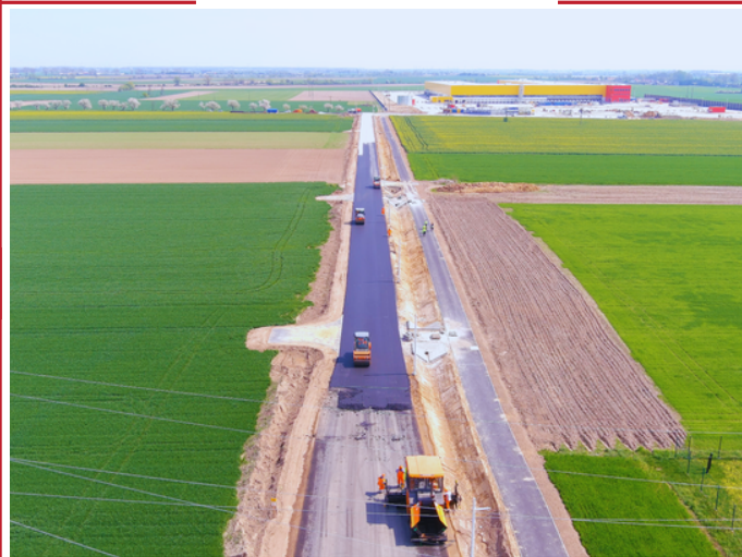
Budowa ul. Stachowskiej - etap II
